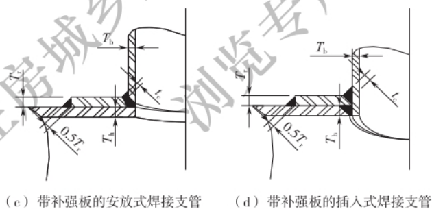
(c) 带补强板的安放式焊接支管
